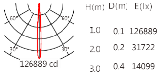
XP-E2 7° 3000K
