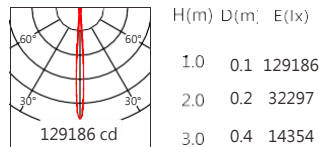
XP-E2 7° 3500K
