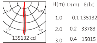
XP-E2 7° 4000K
