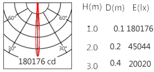
XP-E2 7° 4000K
