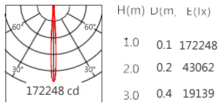
XP-E2 7° 3500K
