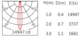
CMU1013 15° 3000K
