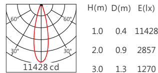
CMB1825 24° 3000K
