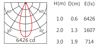
CMB1825 36° 3000K
