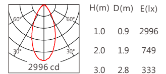
CMB1825 55° 4000K
