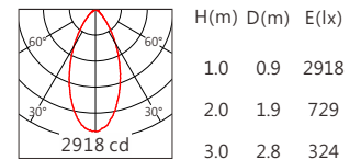
CMB1825 55° 3000K
