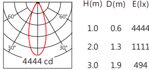
JR-5050 45° 3000K
