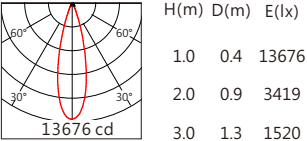
CMB1825 24° 4000K
