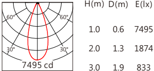
CMB1825 36° 3000K
