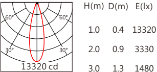
CMB1825 24° 3000K
