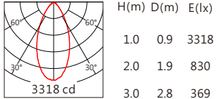
CMB1825 55° 4000K
