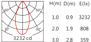
CMB1825 55° 3000K
