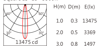
Square ES 15° 3500K
