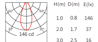
3535 45° RGBW ( 4000K )
