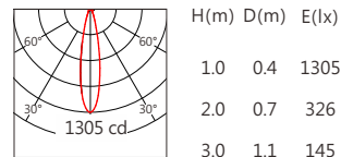
3535 20° RGBW ( 4000K )
