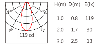
3535 45° RGBW ( 3000K )
