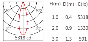
COB CMU 24° 4000K
