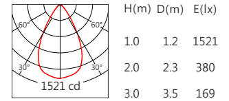
COB CMU 60° 4000K
