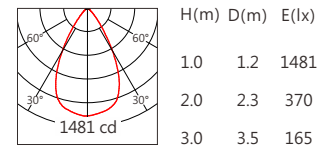
COB CMU 60° 3000K
