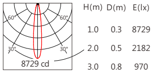
COB CMU 15° 4000K
