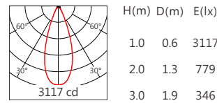
COB CMU 36° 3000K
