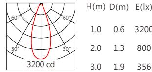
COB CMU 36° 4000K
