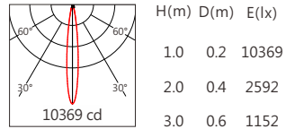
3535 12° RGBW(4000K)
