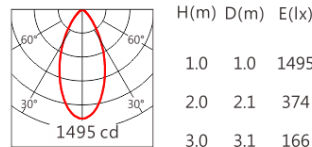
3535 55° RGBW(3000K)
