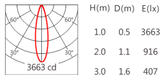
3535 30° RGBW(3000K)
