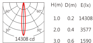
3535 12° RGBW(3000K)
